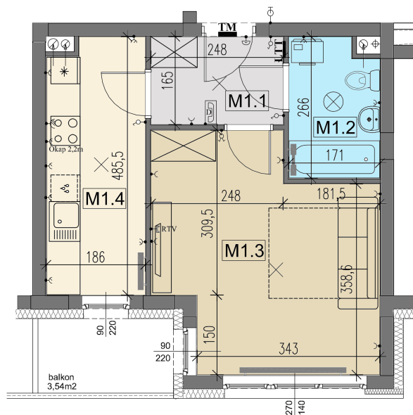
RZUT MIESZKANIA
