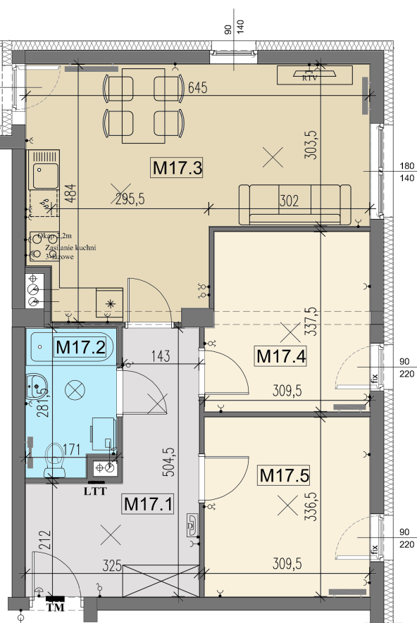
RZUT MIESZKANIA
