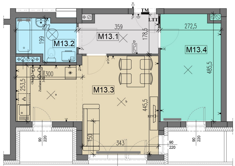
RZUT MIESZKANIA
