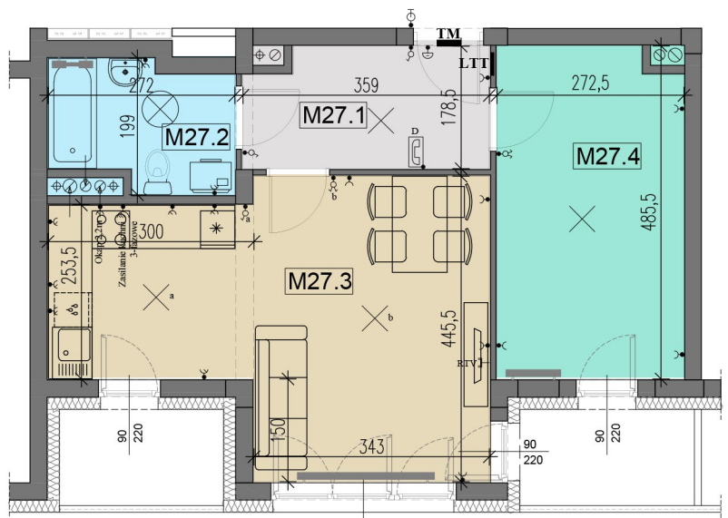
RZUT MIESZKANIA
