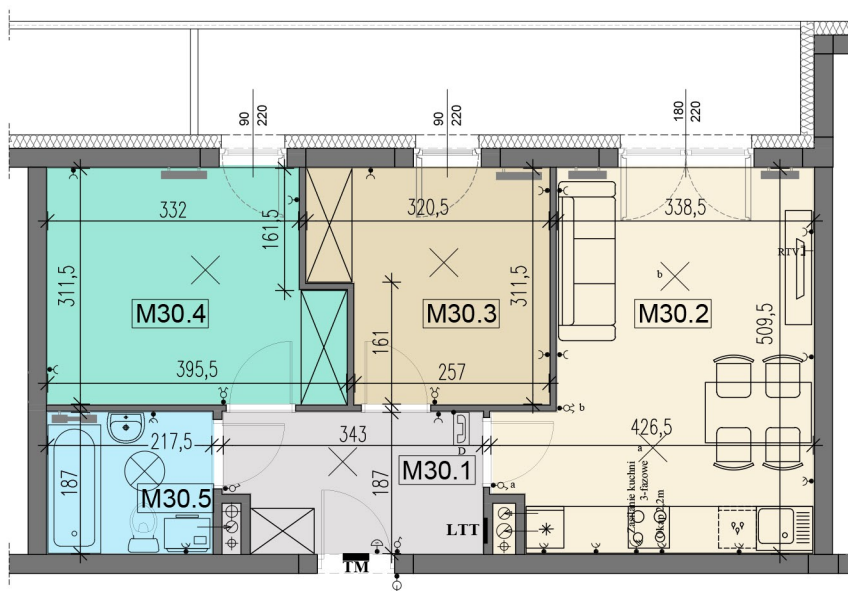
RZUT MIESZKANIA
