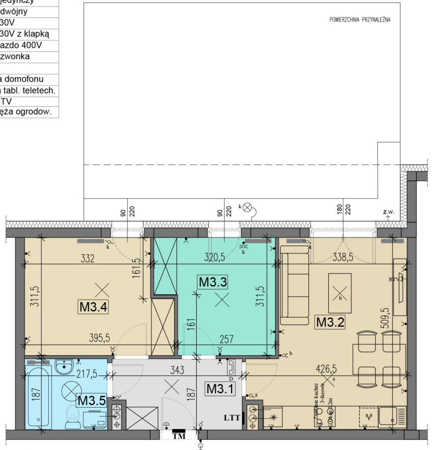
RZUT MIESZKANIA
