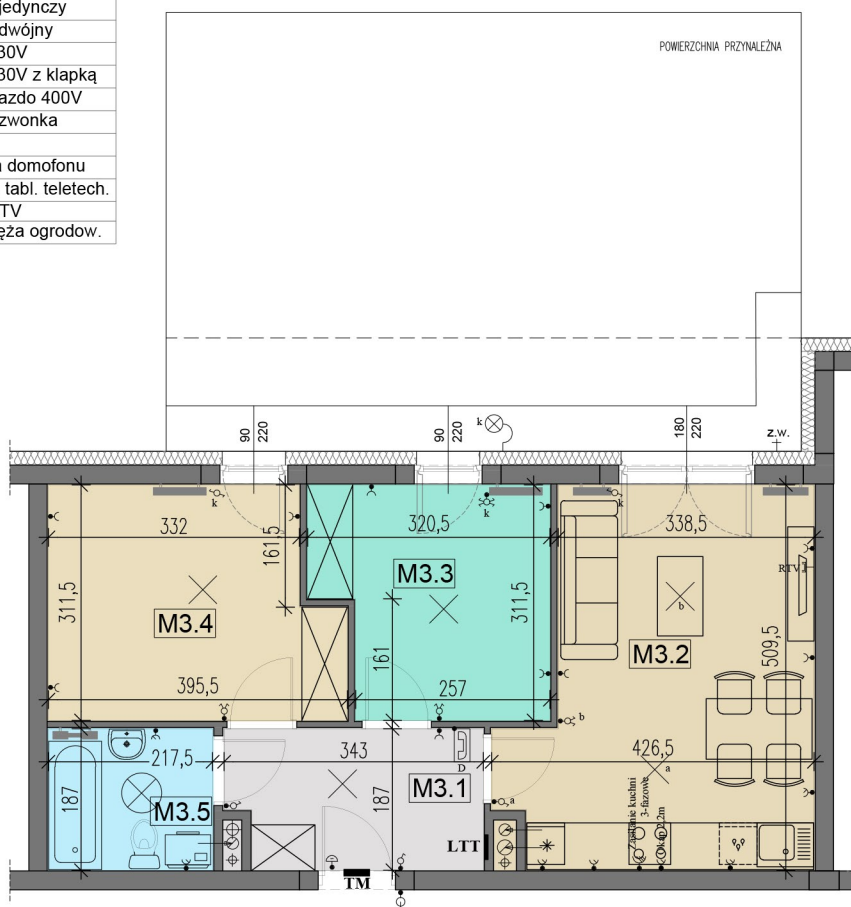
RZUT MIESZKANIA
